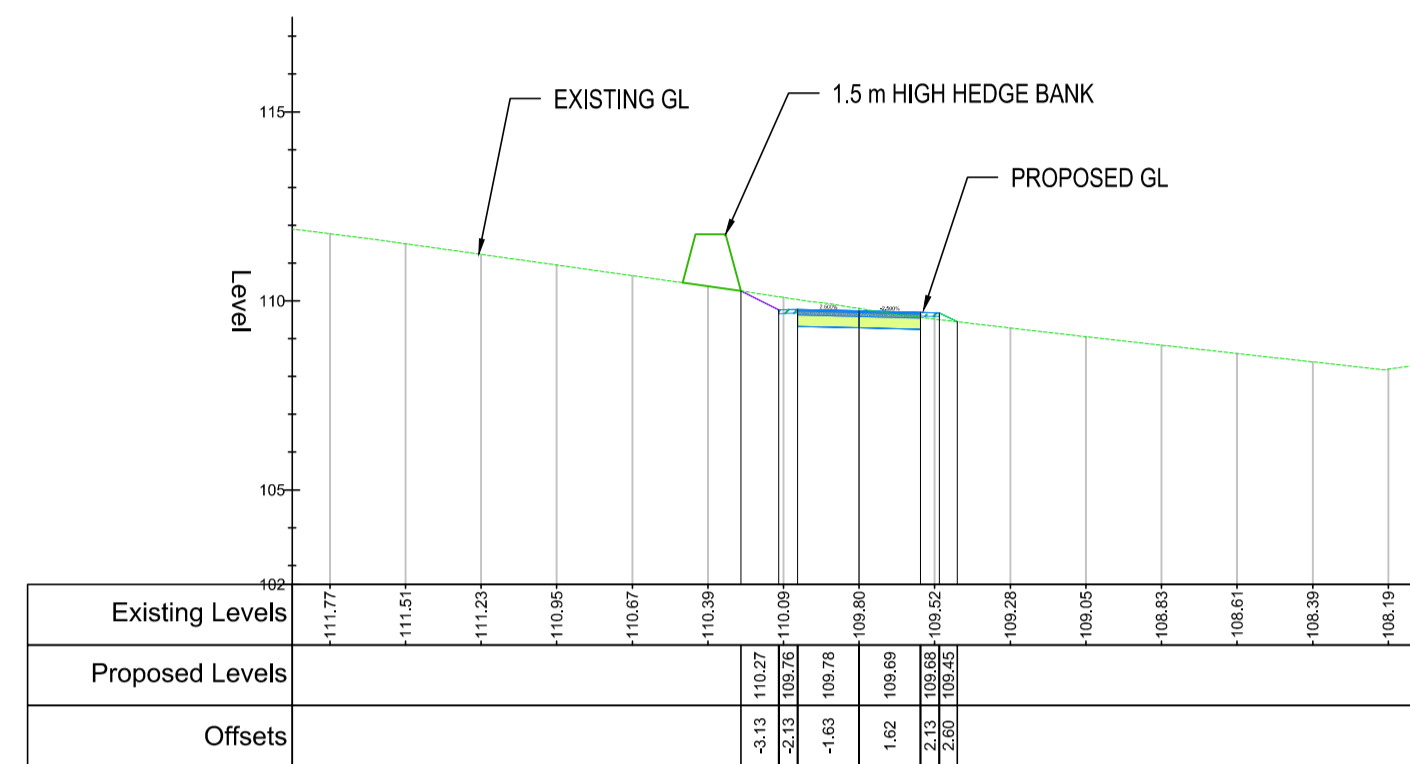
CHAINAGE 250.000 SCALE: H 1:200,V 1:200.
